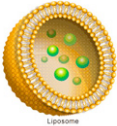
Liposome
